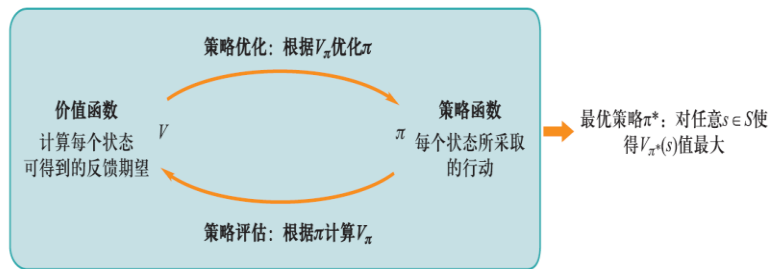
图 6.7 基于通用策略迭代学习最优策略的模式
