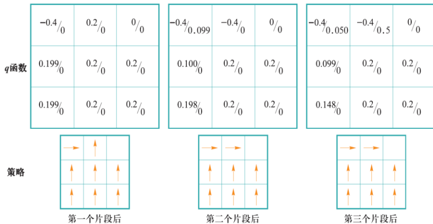
图 6.11 Q 学习执行三个片段的过程
