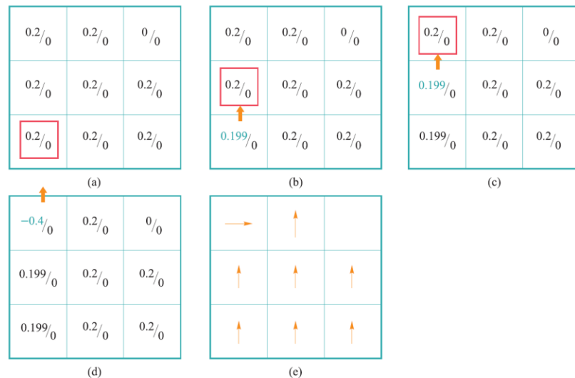
图 6.10 Q 学习的一个片段的执行过程
